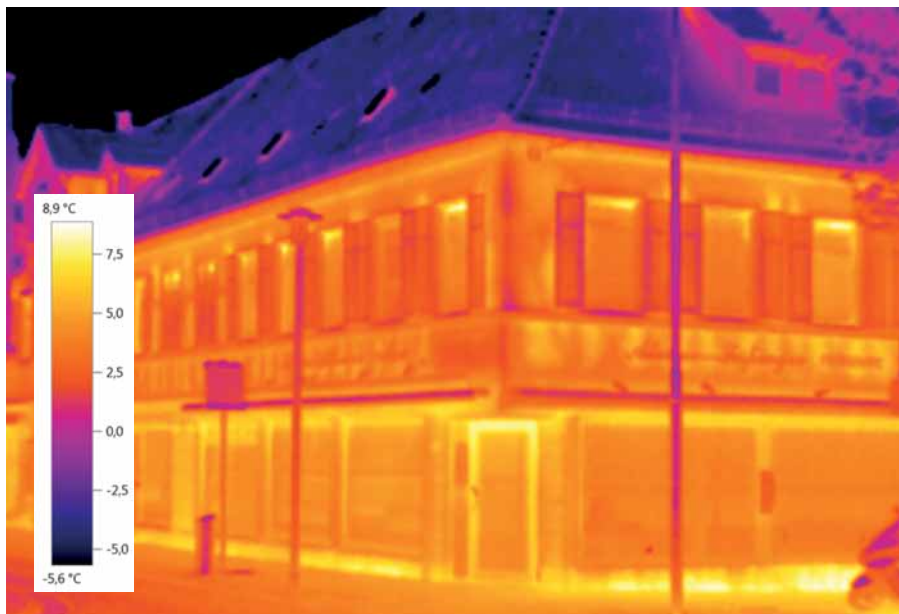
Thermographiaufnahmen zeigen energetische Schwachstellen von Gebäuden.
