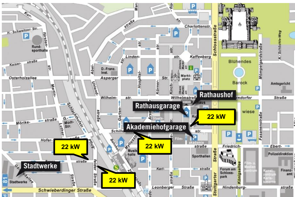
Übersichtsplan Standorte Ladestationen
